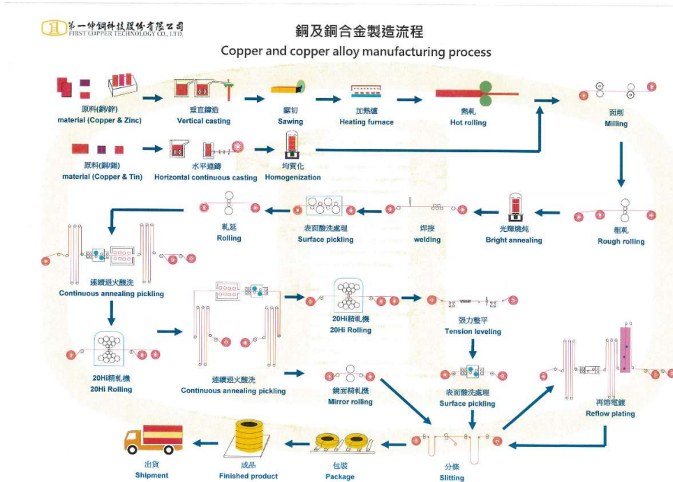
圖 1 第一伸銅科技股份有限公司產品製程
